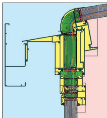
Uf-Berechnung für Profile in Anlehnung an DIN EN ISO 10077-2. Berechnungsmodell (Ausschnitt) mit 52 mm Kalibrierpaneel in Dach und Fenster (Isothermen bei 0°C Außentemperatur).
